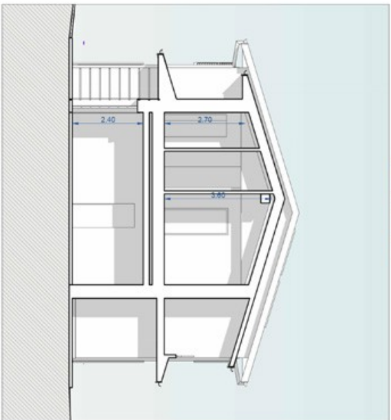
Sezione B-B
