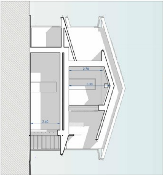
Sezione C-C
